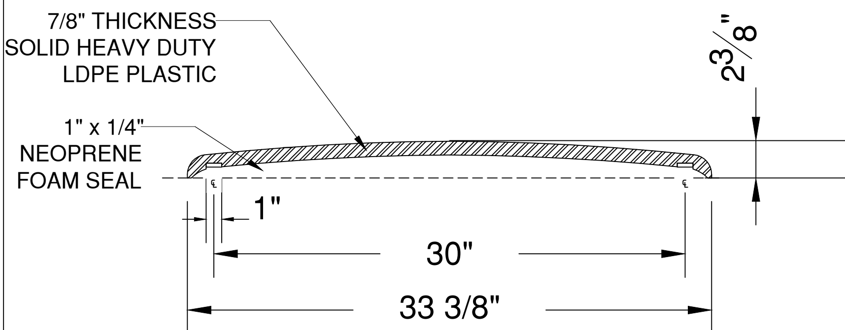
SECTION A-A
